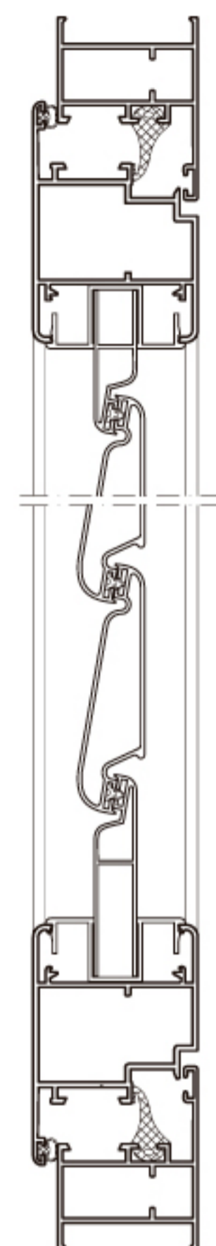
Sección característica
